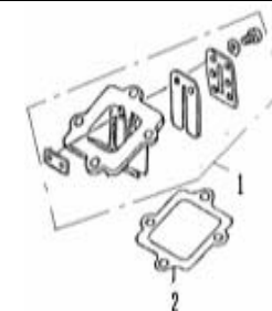
E12 REED VALVE ASSY
