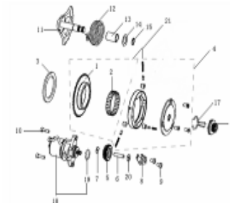
E12 REED VALVE ASSY
