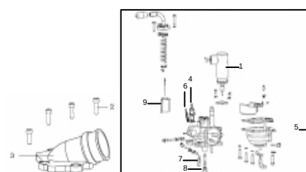
E14 CARBURETOR ASSY
