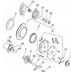
E11 MAGNETO ASSY
