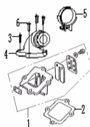
E10 REED VALVE ASSY
