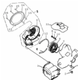
E10 REED VALVE ASSY
