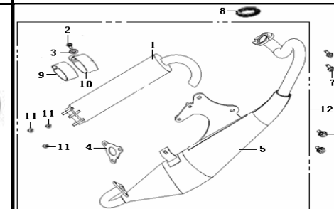
F05-2 RACING-MUFFLER
