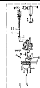
E12 CARBURETOR ASSY
