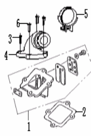
E10 REED VALVE ASSY
