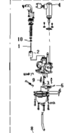
E12 CARBURETOR ASSY
