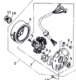
E11 MAGNETO ASSY
