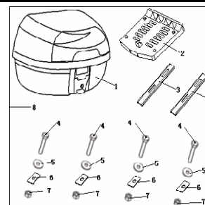
F27 TOP CASE
