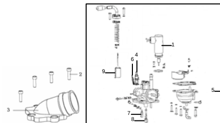
E14 CARBURETOR ASSY
