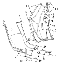
F17 LEG SHIELD
